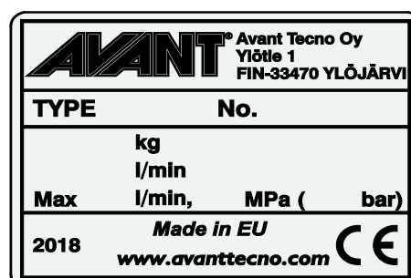
Arbetsredskapets typskylt A417984 / A417990 / A418023
