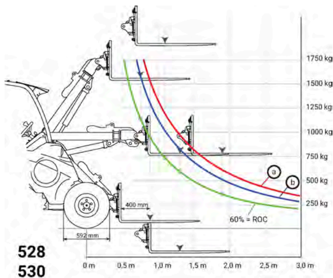
Diagrama de carga < Model3> e 530
