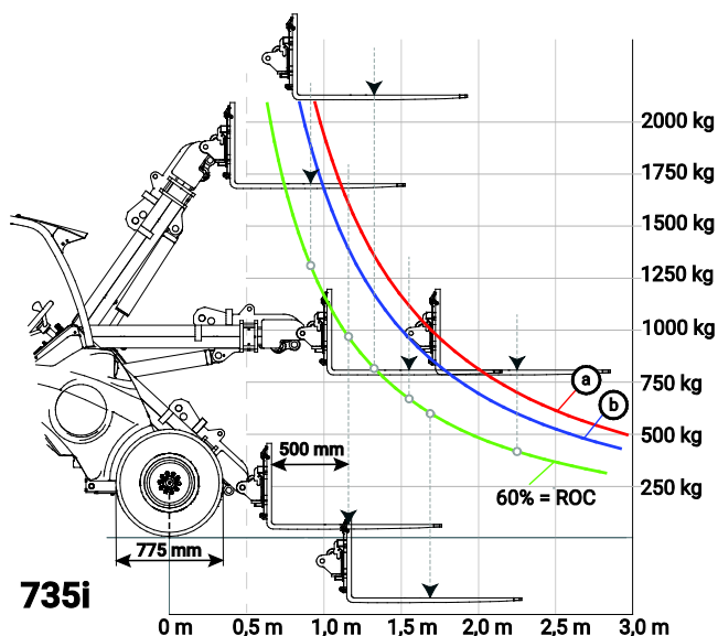
Wykres krzywej obciążenia 735i
