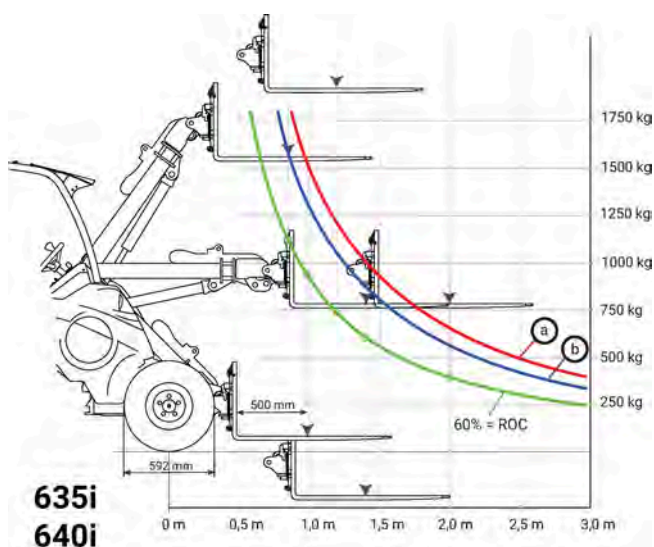
Wykres krzywej obciążenia 635i/640i
