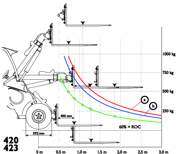
Belastningsdiagram 420
