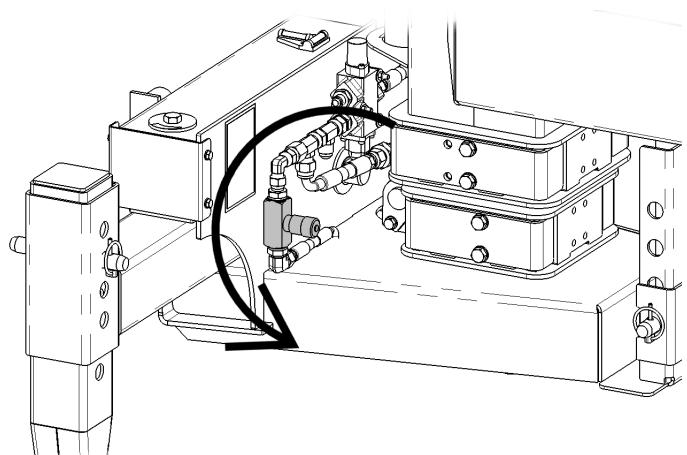
Nooddaalklep bij de snelkoppelingsplaat
