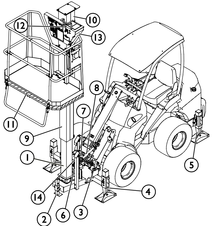
Afbeelding 3 - Hoofdcomponenten van de hoogwerker
