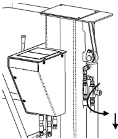
Nooddaalklep op het platform
