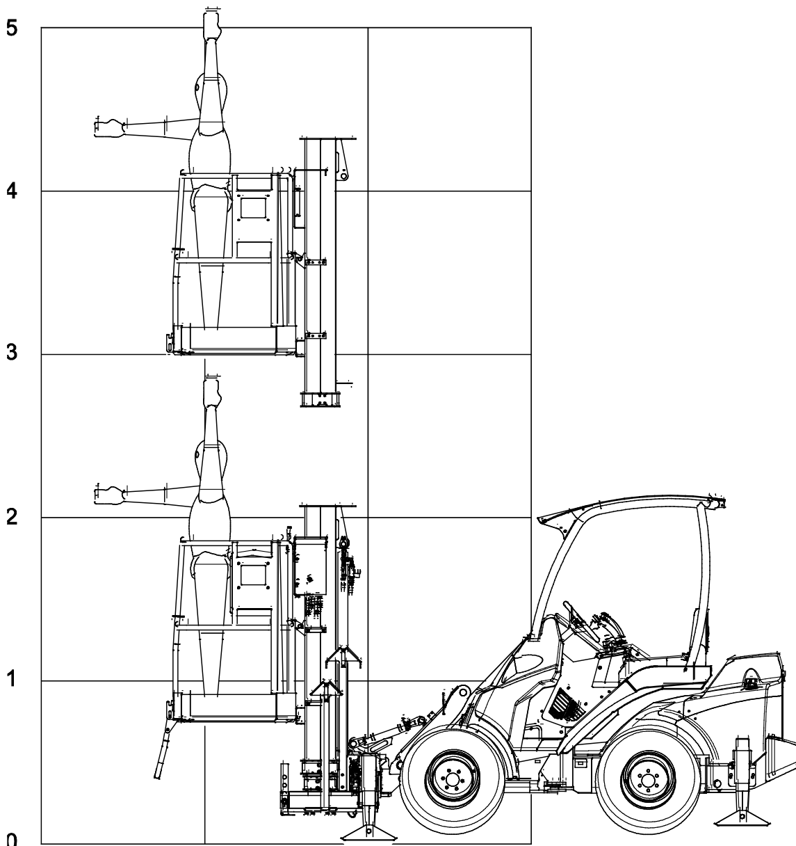
Afbeelding 4 - Leguan 50-hoogwerker vluchtgrafiek
