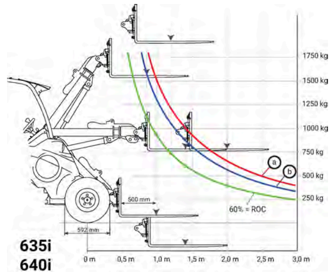
Diagramma di carico 635i/640i
