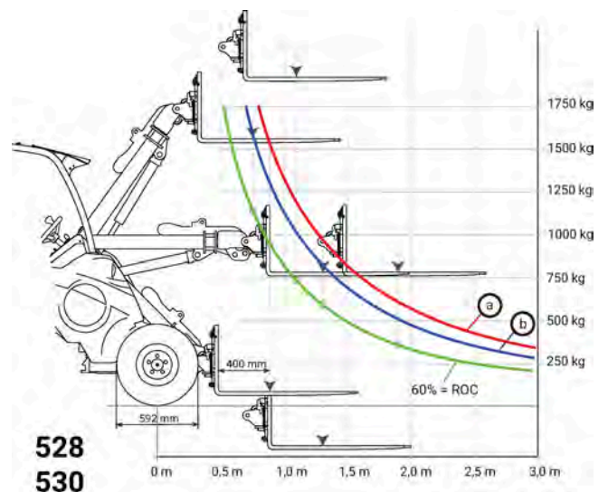
Diagramme de charge 528 et 530
