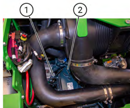
Avant 528 et Avant 530
