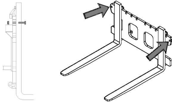
3C. Pernos de sujeción del brazo de la horquilla
