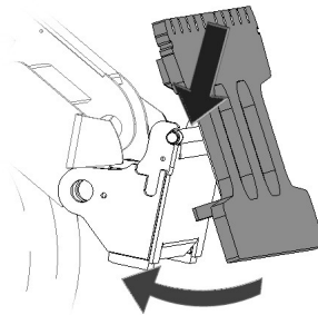
1. Fijación y bloqueo del chasis de la horquilla para palés a la cargadora
