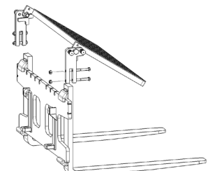
3B. Marco trasero plegable
